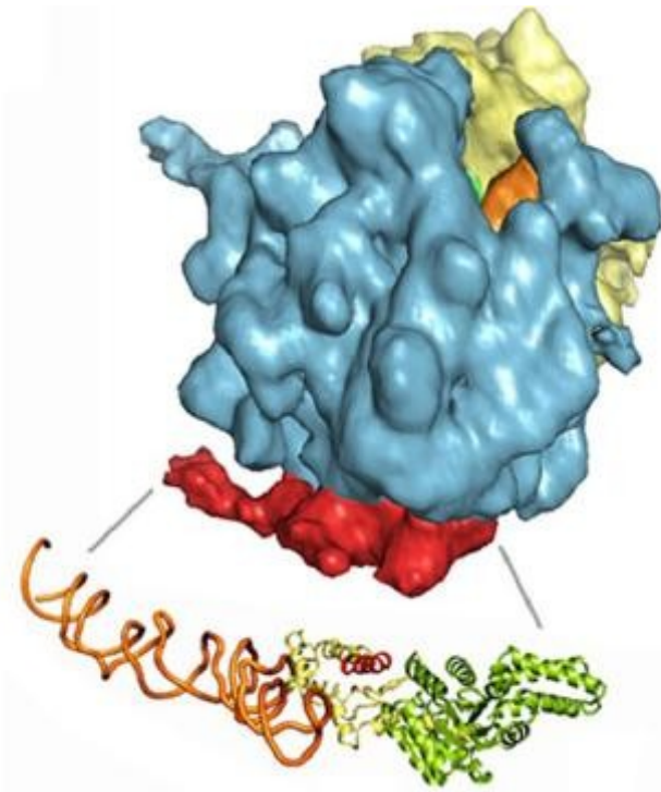
Beispiel für einen Multiprotein Komplex: SRP-Komplex, wie er an das Ribosom gebunden vorliegt. Rekonstruktion nach cryoelektronenmikroskopischen Aufnahmen. © Dr. Christine Schaffitzel, EMBL Grenoble
